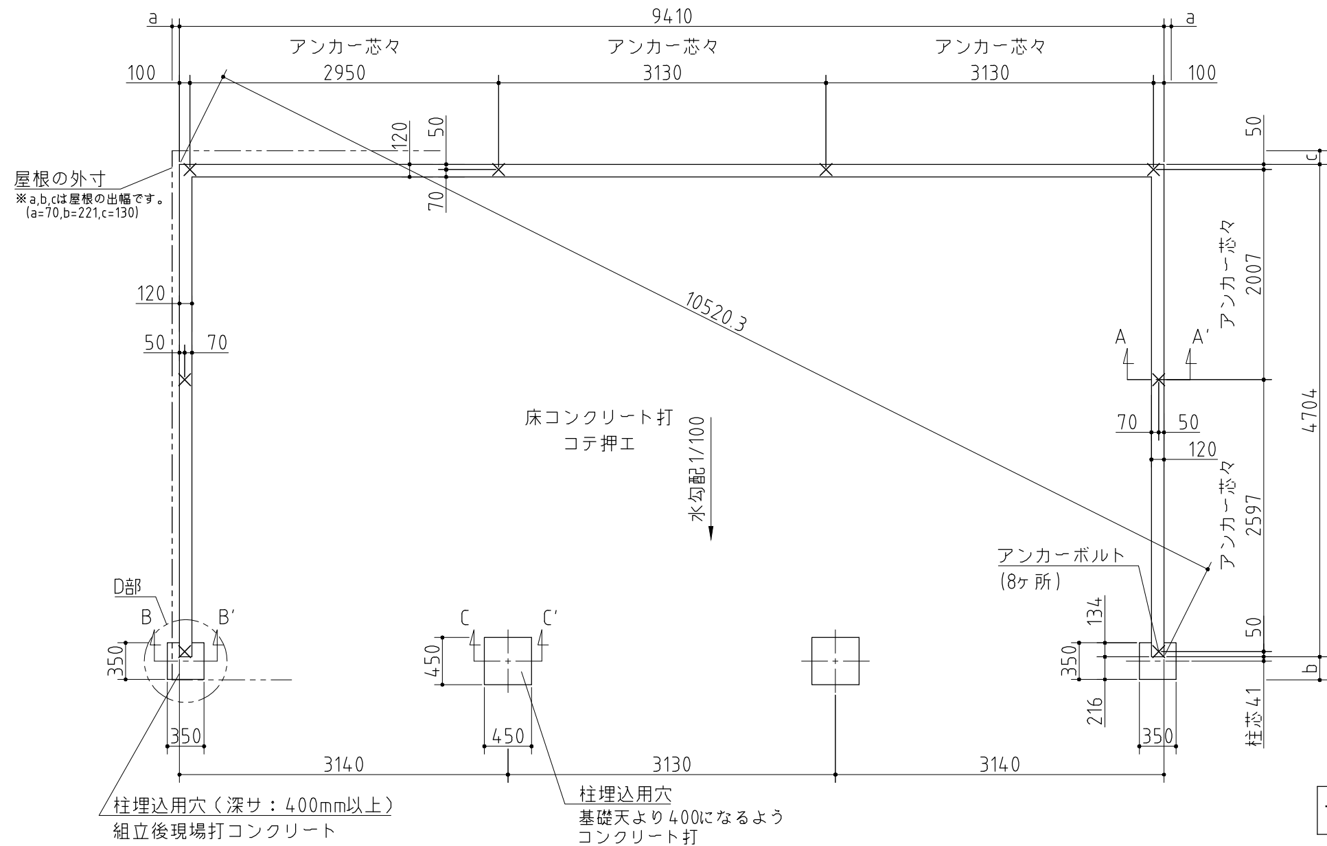
基礎詳細図 S=1/20
